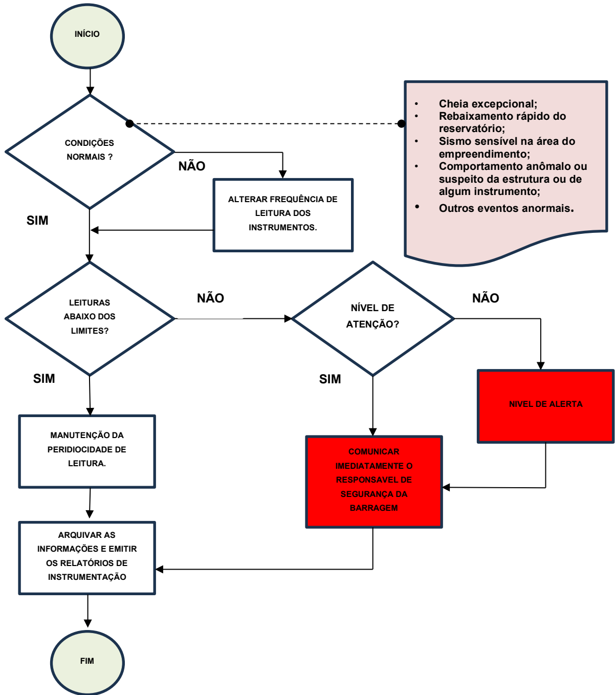
Figura 10: Fluxograma da instrumentação.
