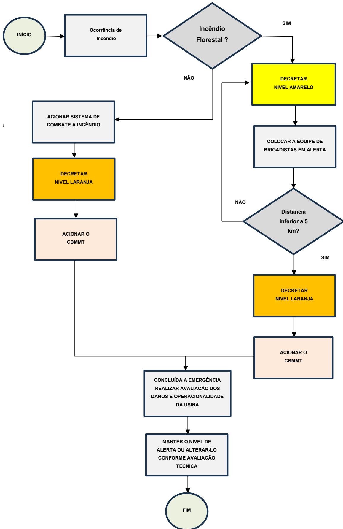
Figura 08: Fluxograma da tomada de decisão de emergência - Incêndio.
