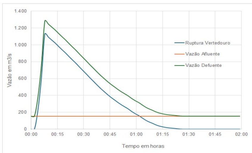
Figura 13: Hidrograma resultante da ruptura da barragem por falha estrutural do Vertedouro - Elevação da Soleira Remanescente = 438,00 m - Vazão Afluente = 153m 3 /s
