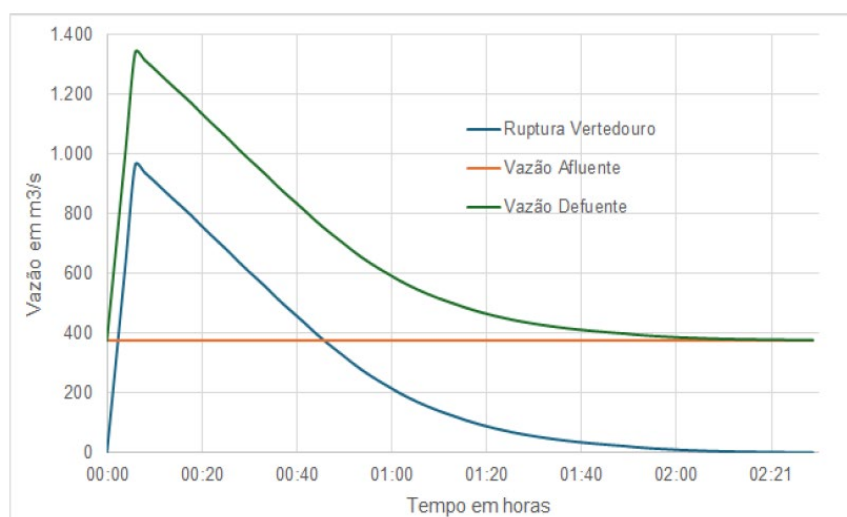
Figura 12: Hidrograma resultante da ruptura da barragem por falha estrutural do Vertedouro - Elevação da Soleira Remanescente = 438,00 m - Vazão Afluente = 375m 3 /s
