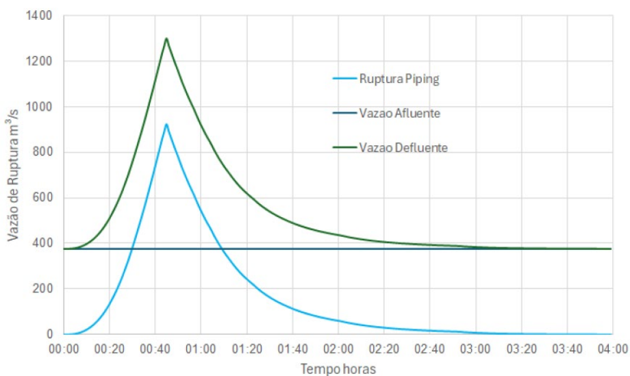
Figura 15: Hidrogramas devido a Ruptura da Barragem por Piping - Cenário 2 - Brecha final na El. 442,00 m e Q decamilenar = 375,0 m 3 /s
