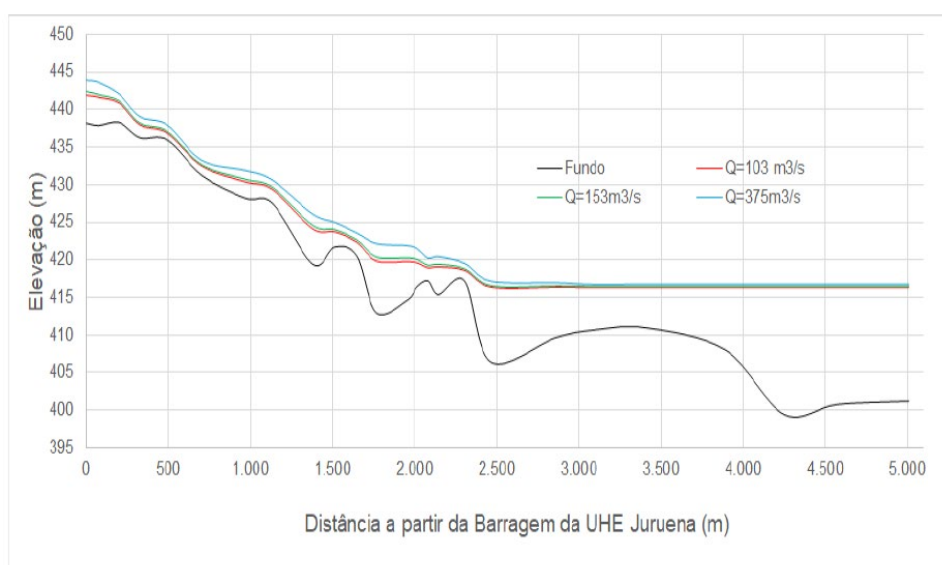
Figura 17: Perfis da Linha D'água em Regime Permanente Rio Juruena entre a UHE Juruena e a PCH Cidezal – Q = 103, 153, 375 m 3 /s.
