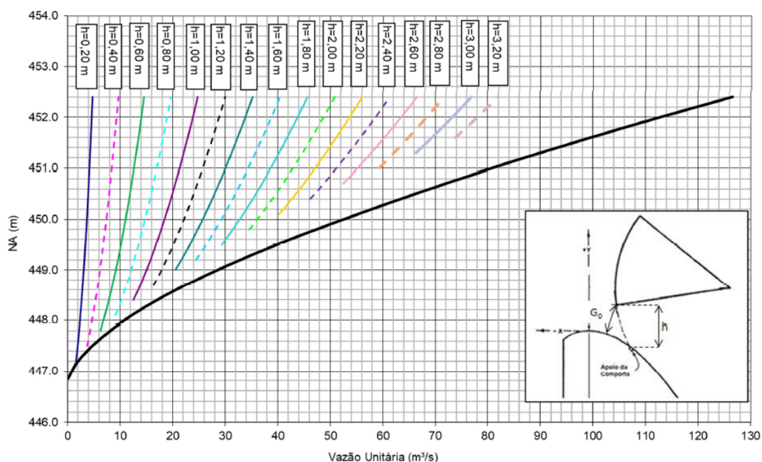
Figura 04: Curva de Abertura Parcial da Comporta x Nível d'Água – Vazão por Um Vão
