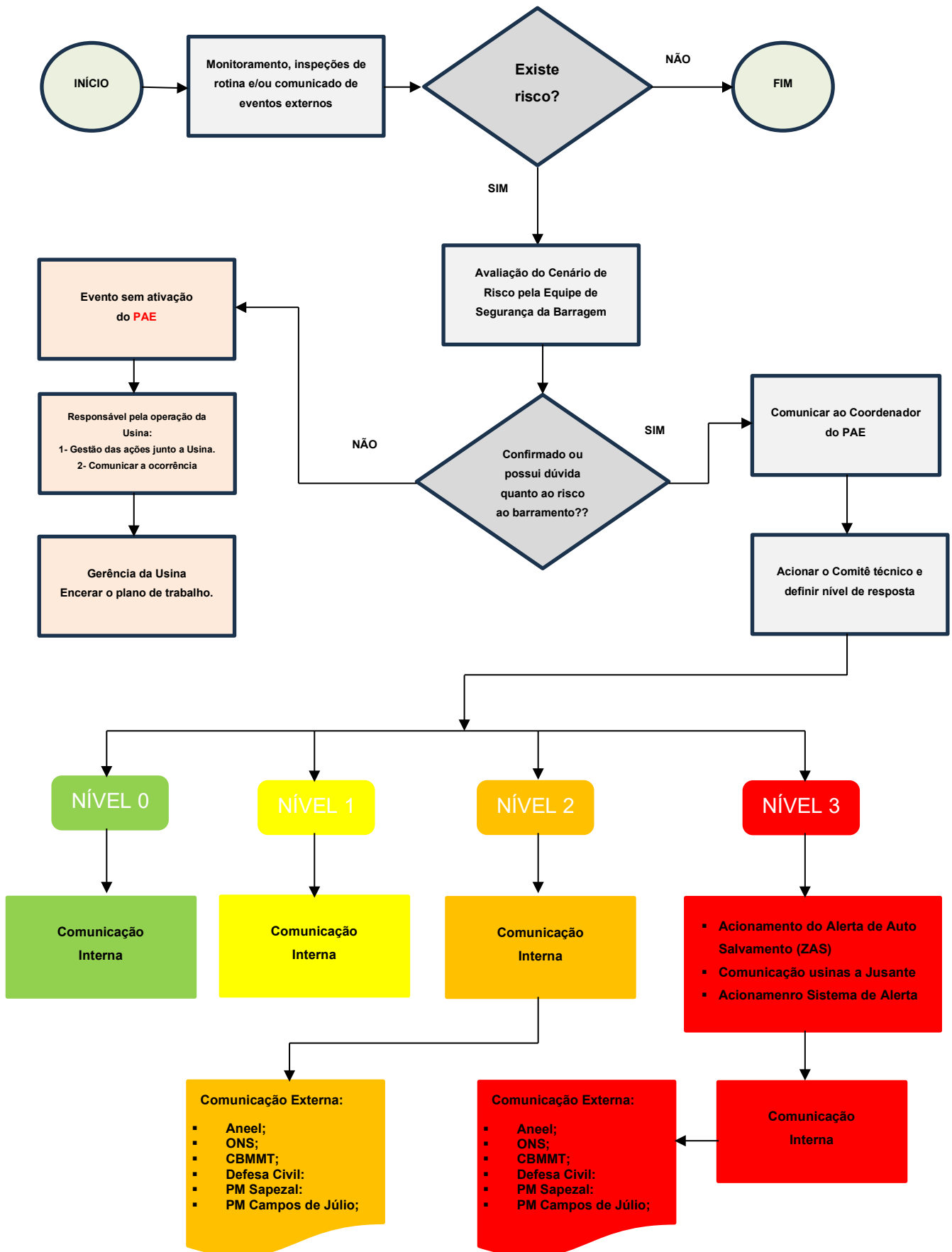
Figura 07: Fluxograma da tomada de decisão de emergência.
