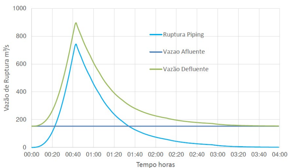
Figura 14: Hidrogramas devido a Ruptura da Barragem por Piping - Cenário 2 - Brecha Final na El. 442,00 m e QMLT = 153,0 m 3 /s
