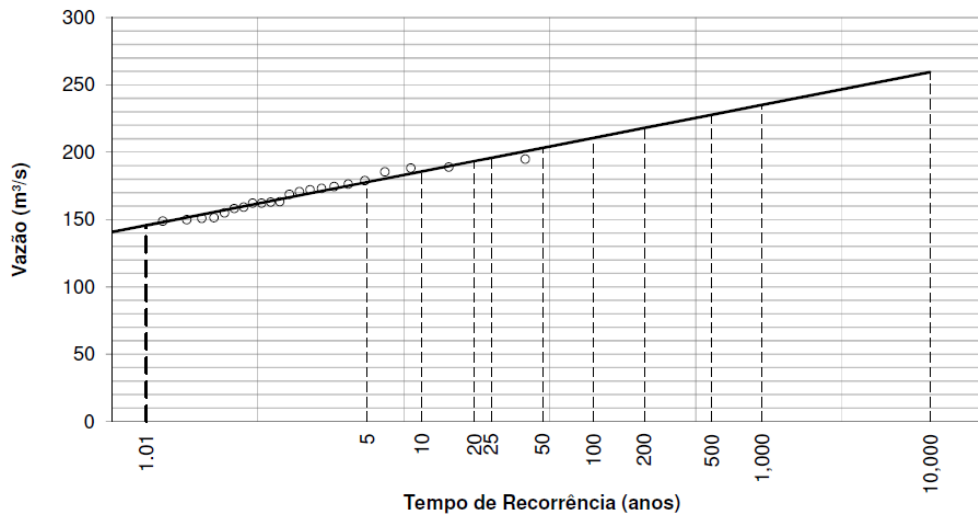
Figura 11: Ajuste da Distribuição de Gumbel às Vazões de Cheia - Rio Juruena em Fazenda Tucunaré - Período: 1995 a 2017
